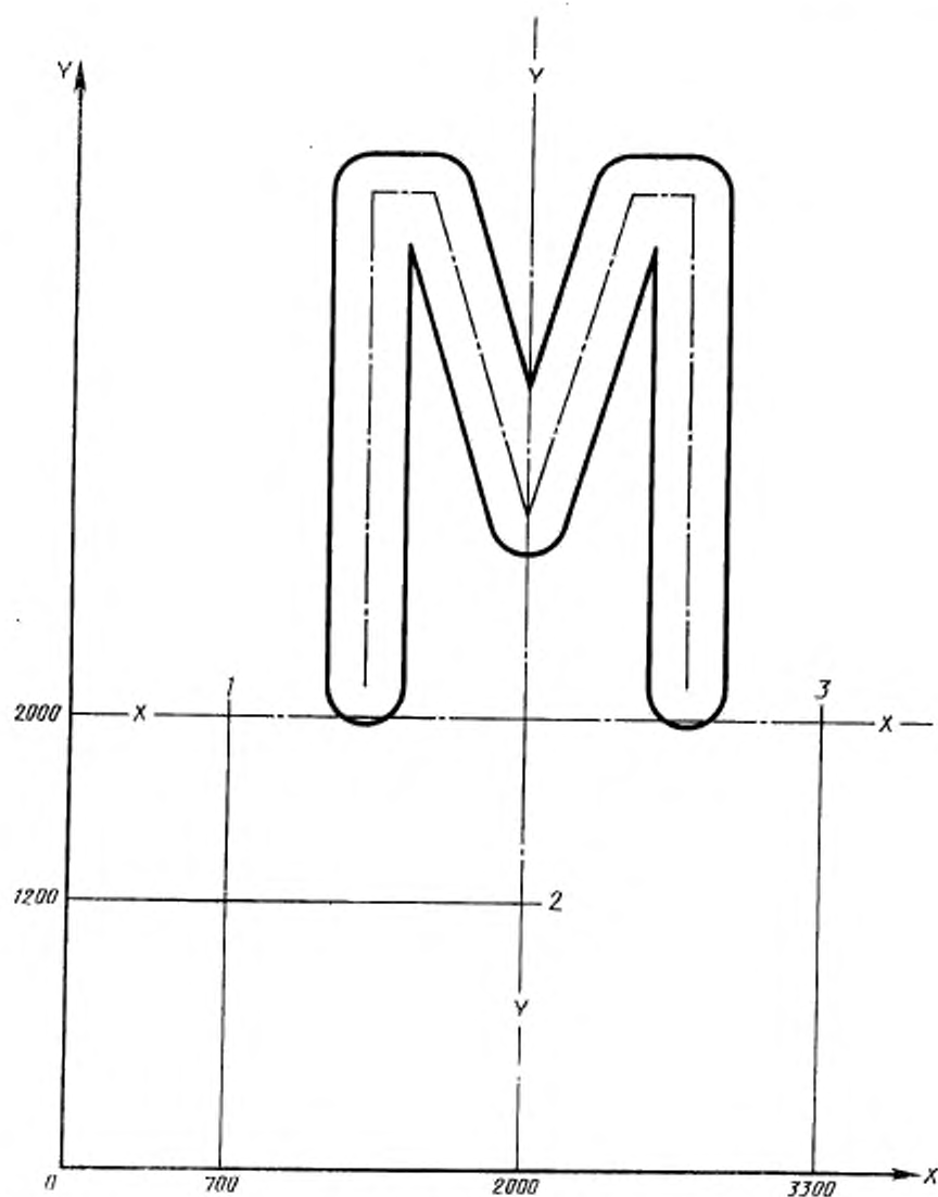
X—горизонтальная базовая линия для шрифта РОС-А; Y—вертикальная базовая линия для шрифта РОС-А
