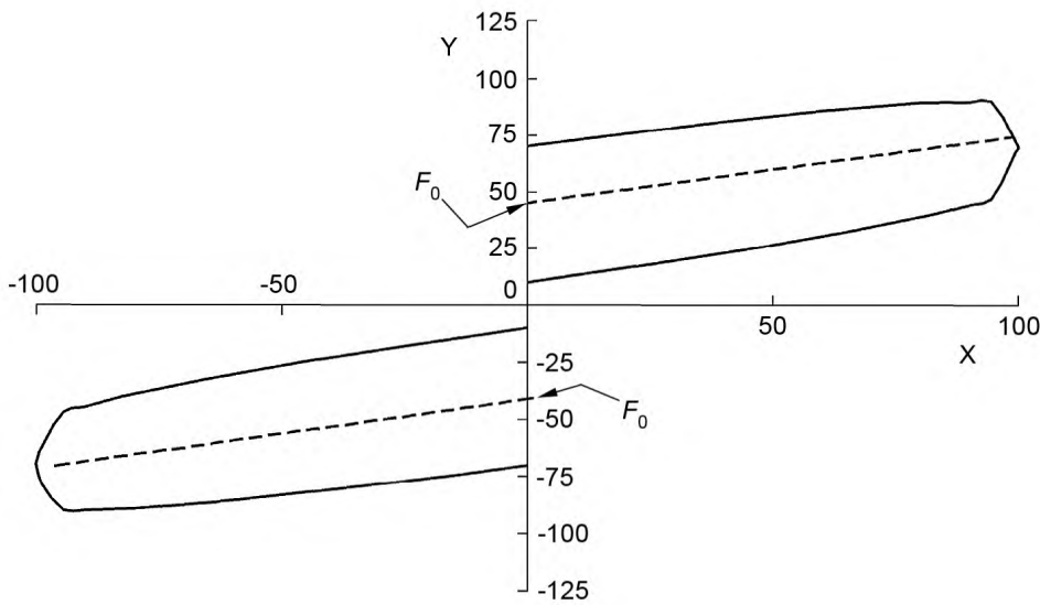
X — нормированное перемещение, %; Y — нормированная сила, %
