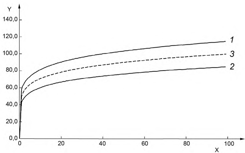
X — нормированная скорость, %; Y — нормированная сила, %; 1 — верхний предел; 2 — нижний предел; 3 — характеристическая кривая зависимости силы от скорости
