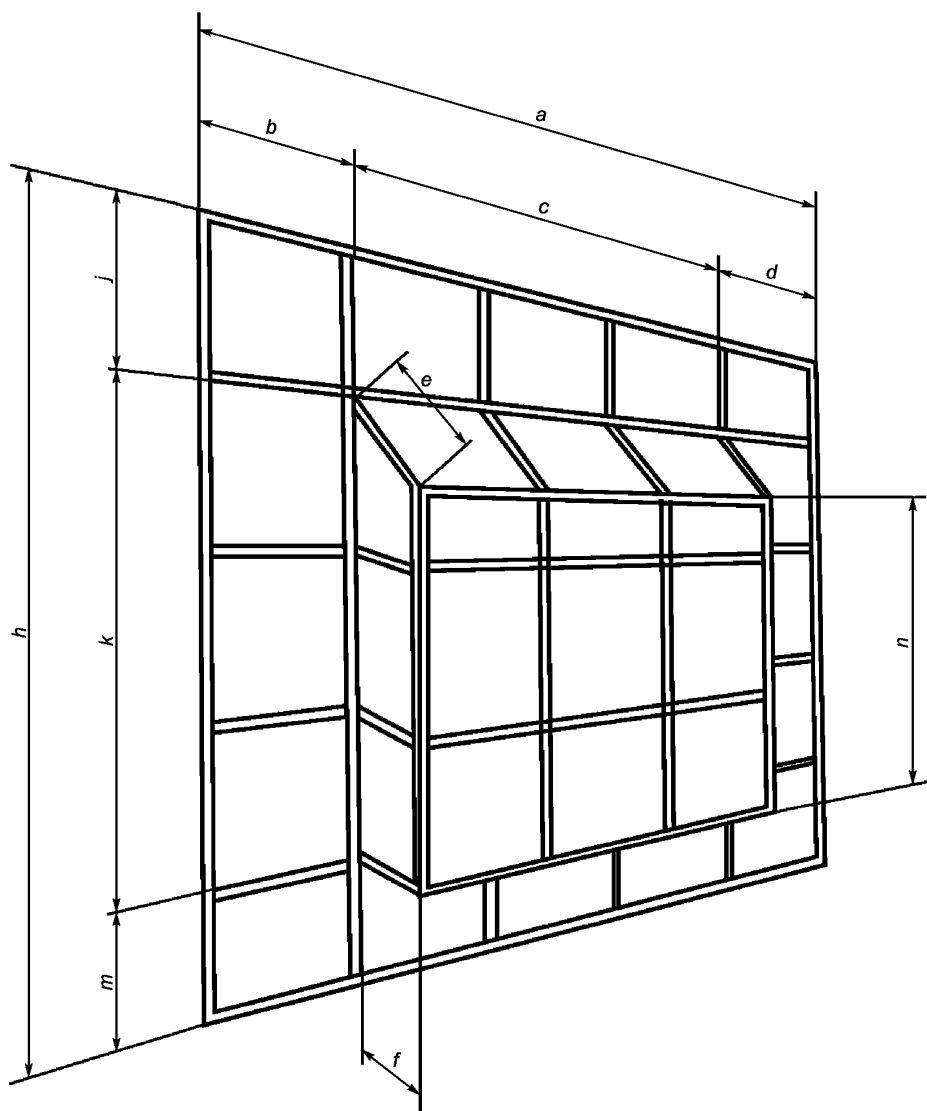
Рисунок 2 — Схема расчета площади испытуемого образца
