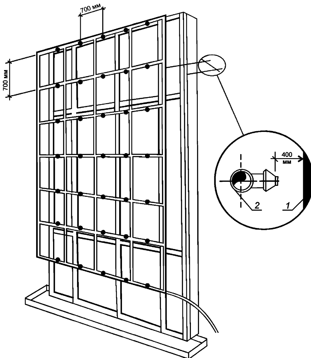
1 — образец для испытаний; 2 — форсунка дождевальной системы
