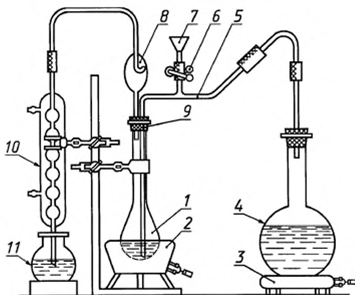
1 — колба Кельдаля; 2 — колбонагреватель; 3 — электролитка; 4 — парообразователь; 5 — соединительная трубка; 6 — зажим; 7 — воронка; 8 — каплеуловитель; 9 — пробка; 10 — холодильник; 11 — приемная колба
